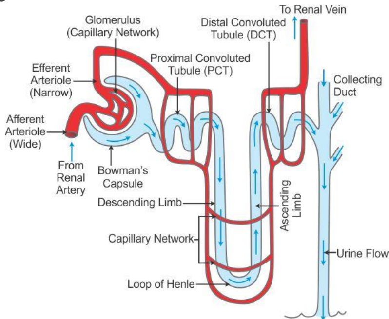
Uriniferous Tubule
