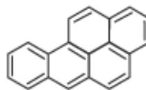
1,2-Benzpyrene
