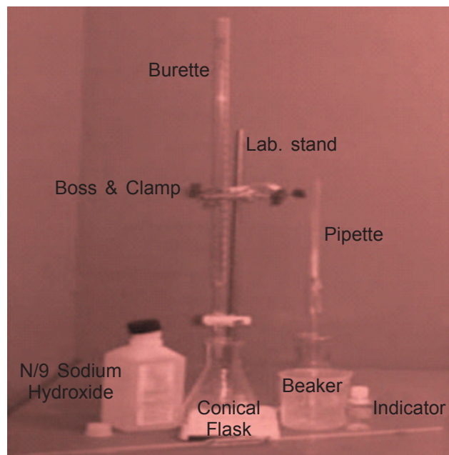
Fig.1.1. Titratable acidity apparatus
