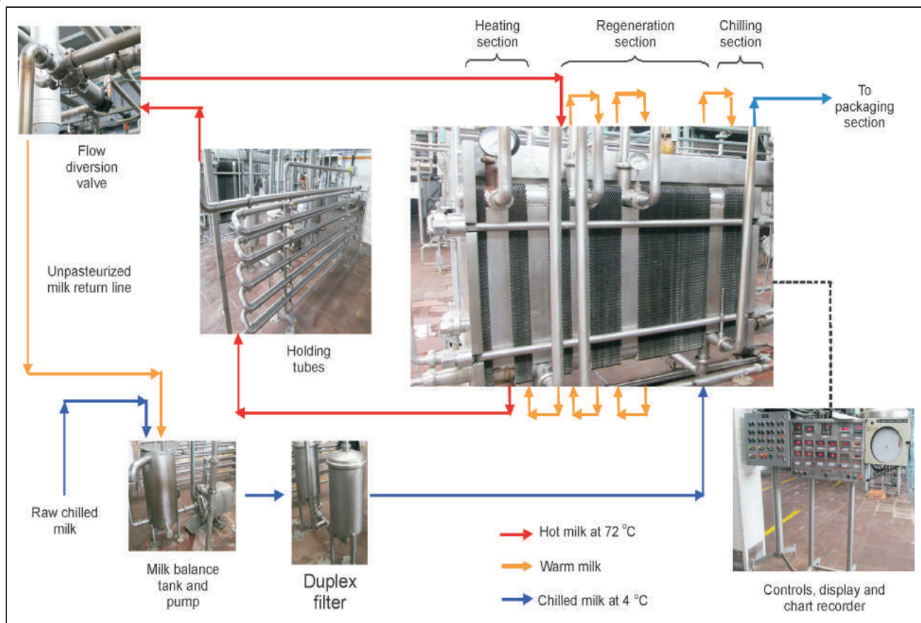
Fig.8.3. HTST Pasteurizer
