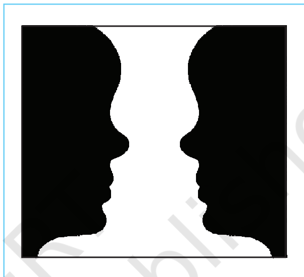
Fig.5.6 : Rubin's Vase
