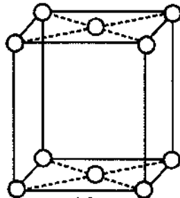
अन्तःकेन्द्रित (bcc)
