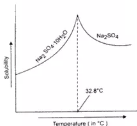
Fig. 6.10: Solubility curve for \text{Na}_2\text{SO}_4 \cdot 10\text{H}_2\text{O} (Glauber's salt)
